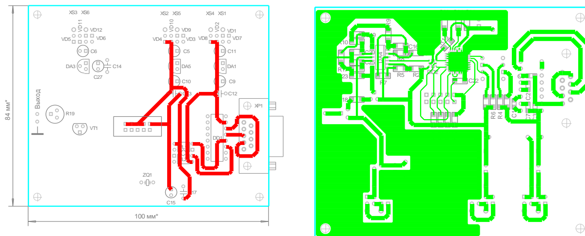
Рисунок 6 – Печатная плата
